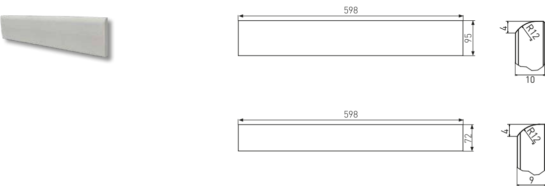
Sockel | skirting plinth | TSASZ... | 598×95×10 mm* TSAS3... | 598×72×9 mm **
